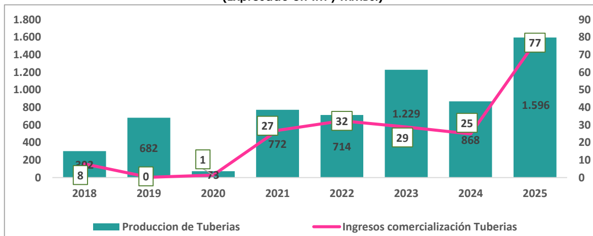
GRÁFICO N°20: PRODUCCIÓN DE TUBERÍAS E INGRESOS POR SU COMERCIALIZACIÓN (Expresado en TM y MMBs.)
