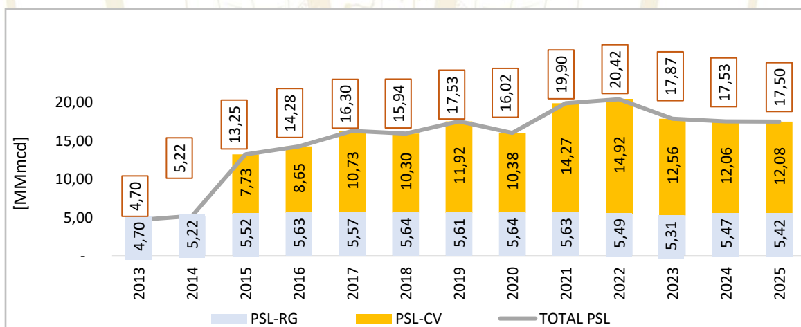
GRÁFICO N° 16 GAS PROCESADO PLANTAS SEPARADORAS DE LÍQUIDOS
