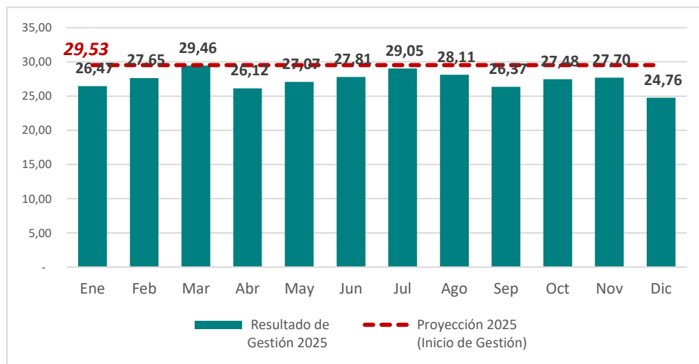
GRÁFICO N° 5. PRODUCCIÓN FISCALIZADA SUJETA A REGALÍAS DE GAS NATURAL en Millones de Metros Cúbicos por Día (MMmcd)
