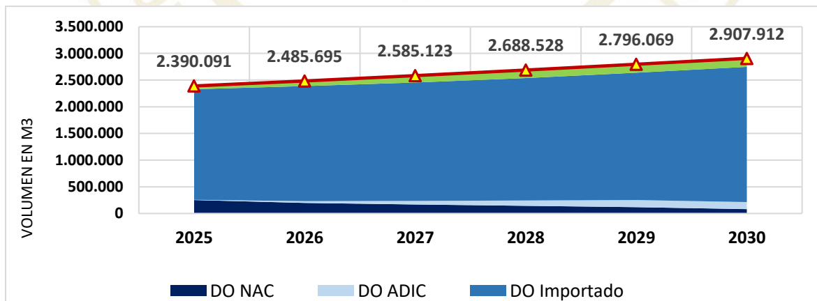
GRÁFICO N°29 BALANCE DE OFERTA Y DEMANDA DE DIÉSEL EN BOLIVIA (En m3)
